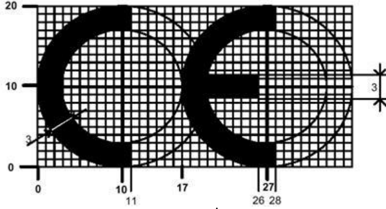
Şekil 3 : CE İşareti
